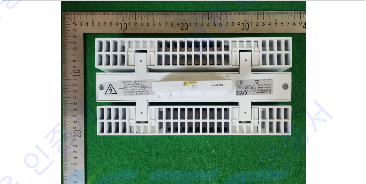
NO. 4 제품옆면
